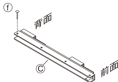
ストッパーピン取り付け位置
