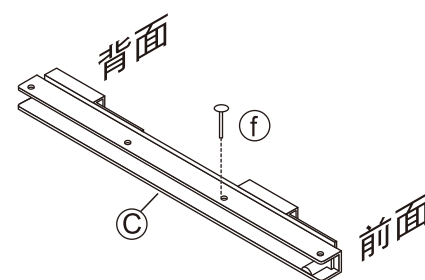
ストッパーピン取り付け位置
